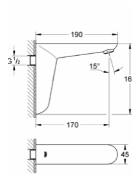
36 274 000 Euroeco Cosmopolitan E
