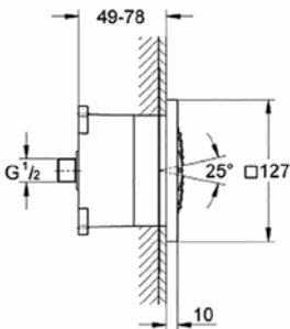
27 251 000 Rainshower® F-Series 5\"/>
