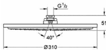
27 477 000 Rainshower® Cosmopolitan 310
