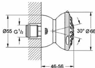
27 067 000 Relaxa 65
