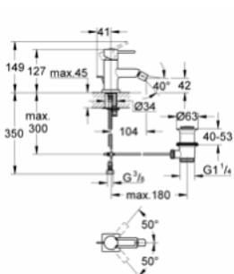
32 147 000 Bidet mixer
