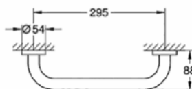
40 421 001 Grip bar 295mm
