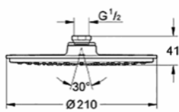
28 368 000 Rainshower® Cosmopolitan 210
