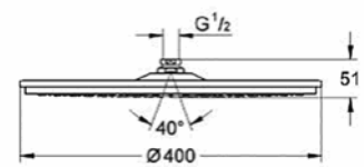
28 778 000 Rainshower® Cosmopolitan 400
