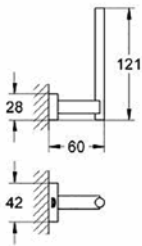
40 623 001 Spare toilet roll holder
