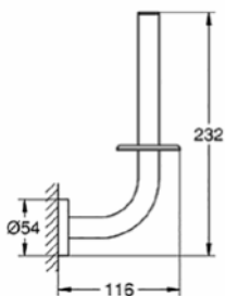
40 385 001 Spare toilet roll holder
