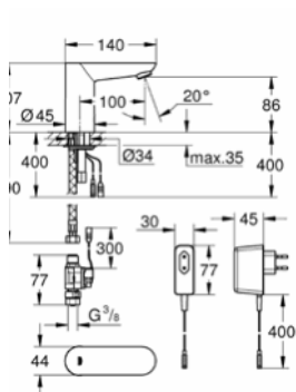
36 269 000 Euroeco Cosmopolitan E
