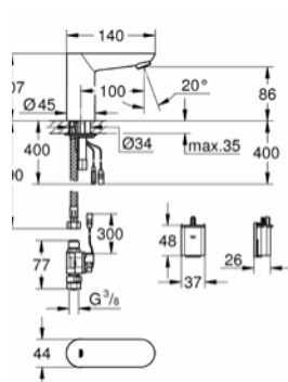
36 271 000 Euroeco Cosmopolitan E
