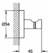
40 364 001 Robe hook
