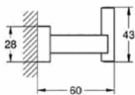
40 511 001 Robe hook
