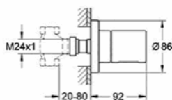
19 470 000 Grohtherm 3000 Cosmopolitan
