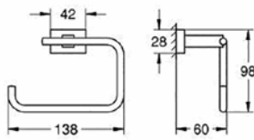
40 507 001 Toilet roll holder
